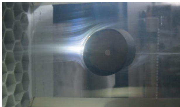
DBDプラズマアクチュエータ による気流制御実験
